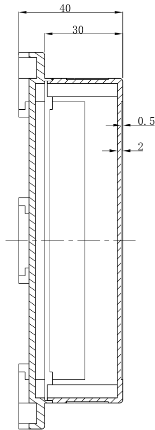
截面 A-A
