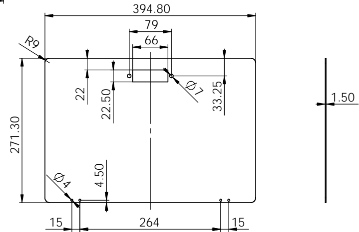
面板尺寸
