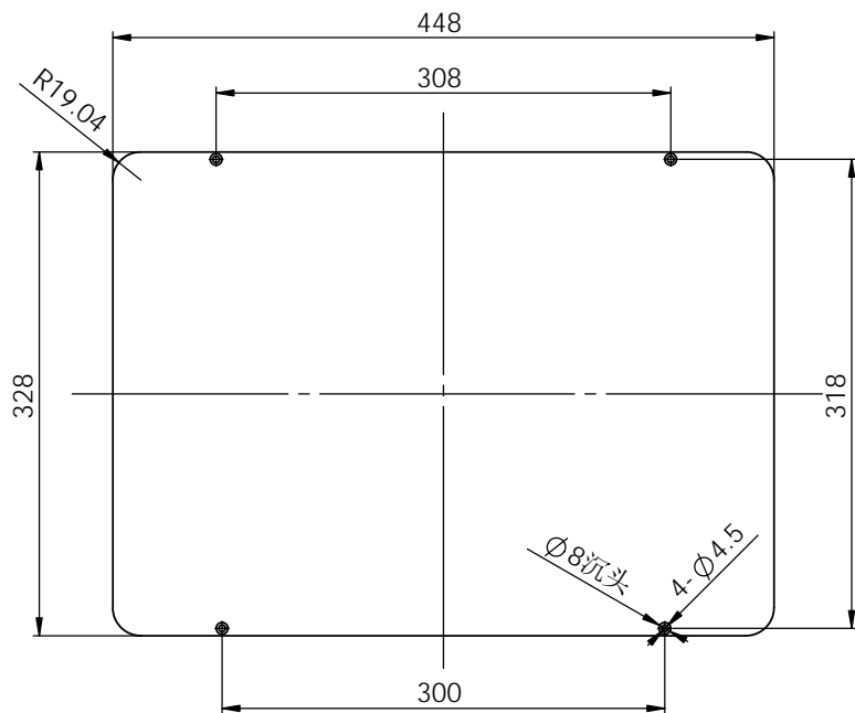
面板尺寸图
