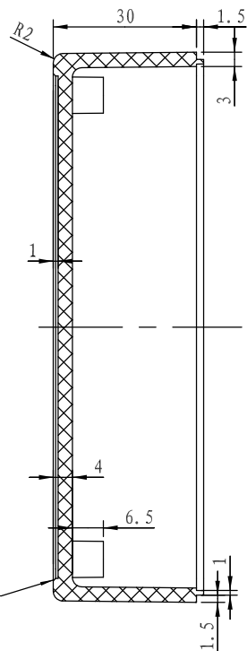
剖面 B-B
