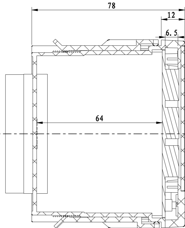
截面 A-A
