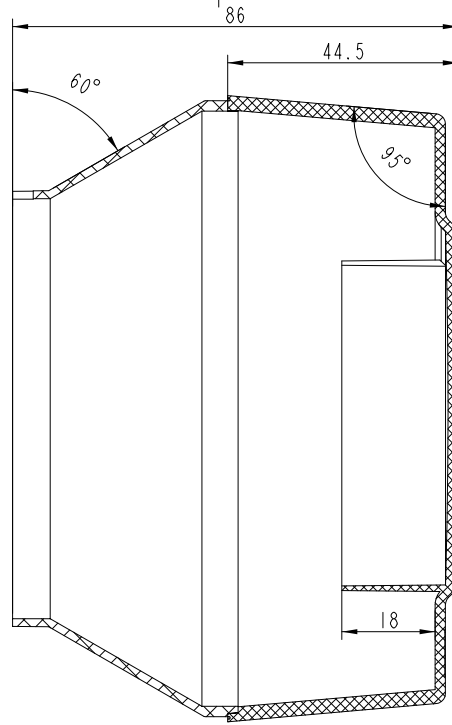
剖面 A-A
