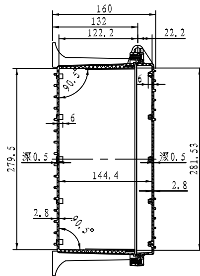
截面 A-A
