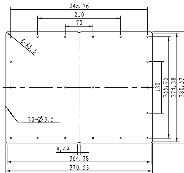
建议PCB尺寸
