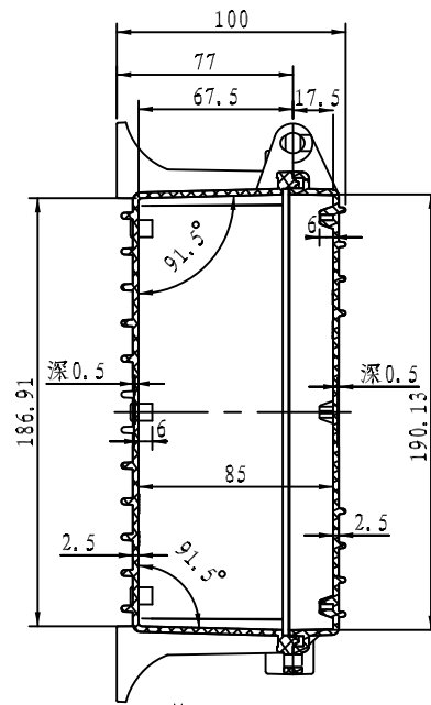
截面 A-A
