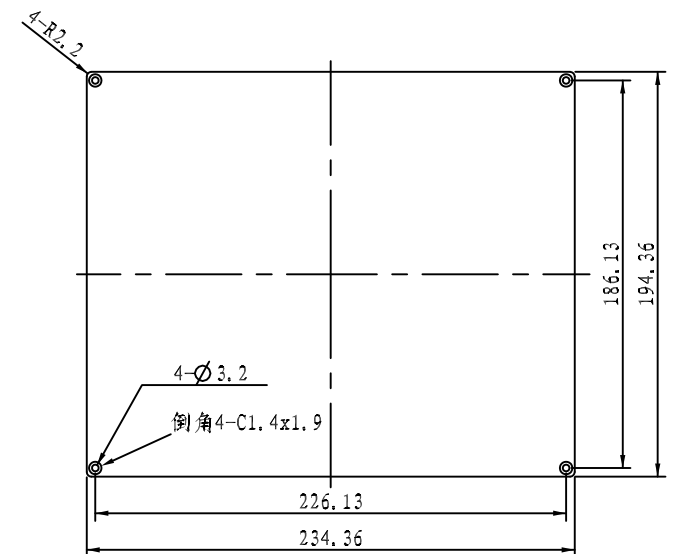
面板
