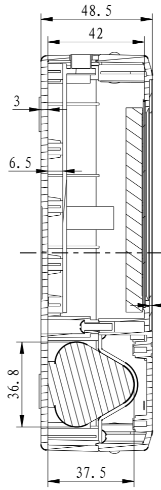
剖面 A-A
