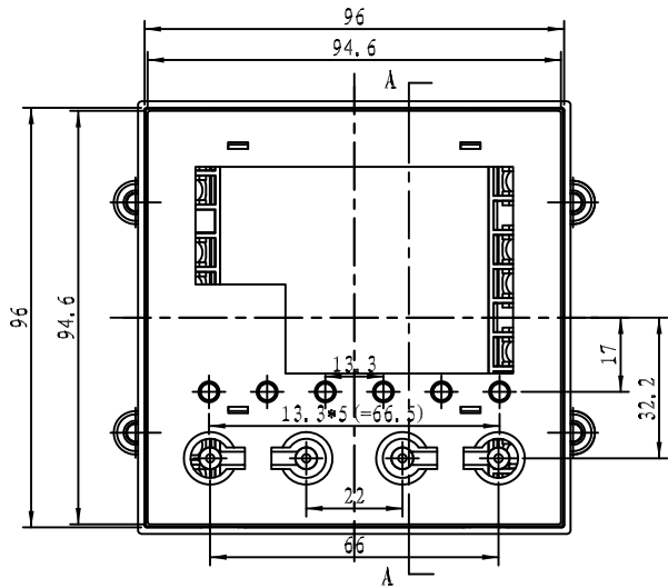
比例 4:5
