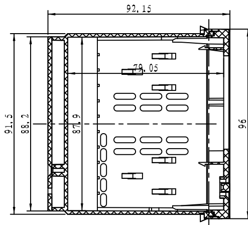
剖面 A-A
