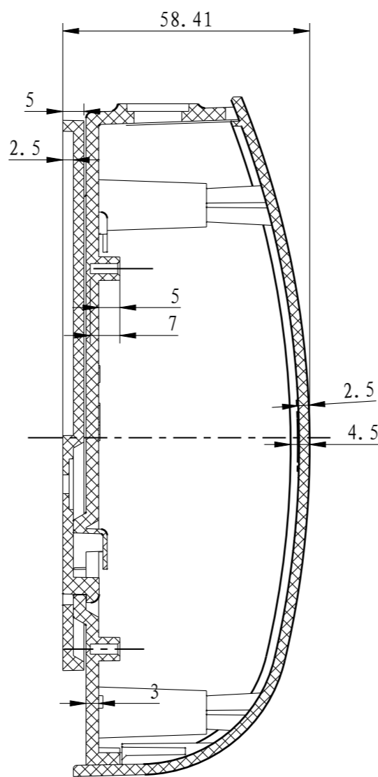
剖面 D-D
