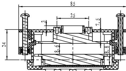
剖面 A-A
