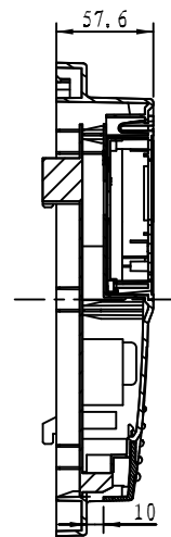
剖面 A-A
