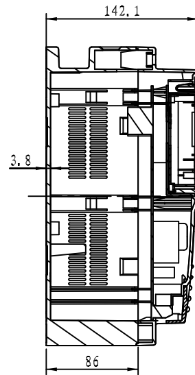
剖面 A-A
