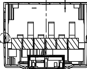
剖面 B-B
