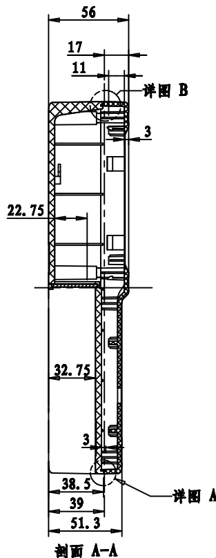
剖面 A-A
