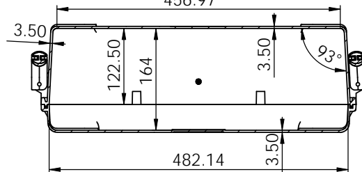
剖面 C-C 456.97
