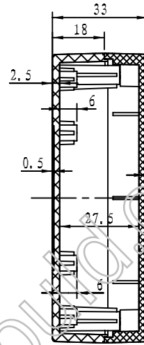
剖面 B-B
