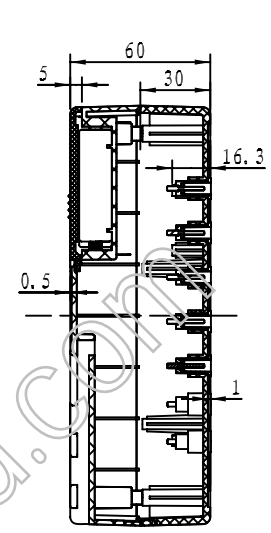
截面 A-A
