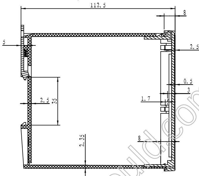
前面 A-A
