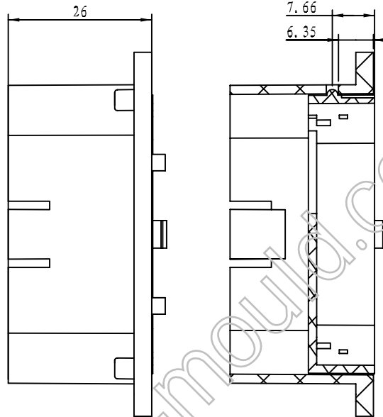
剖面 B-B
