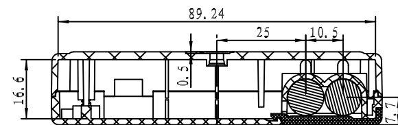
截面 A-A
