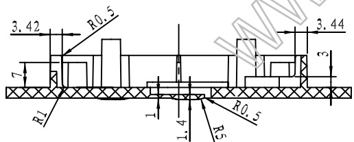
剖面 A-A
