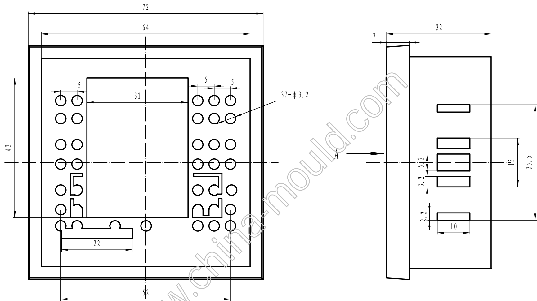
A向视图
