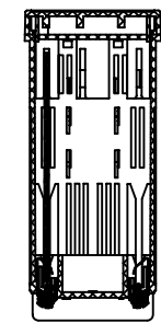
剖面 A-A
