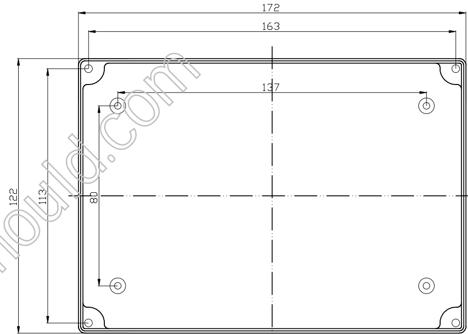
下盖正视图
