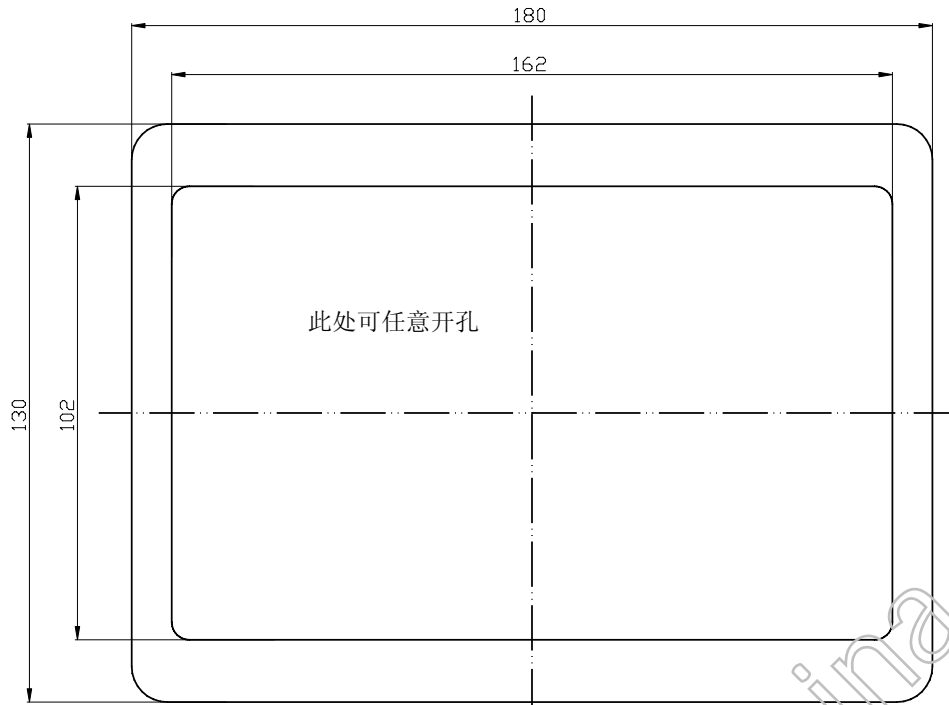
上盖正视图
