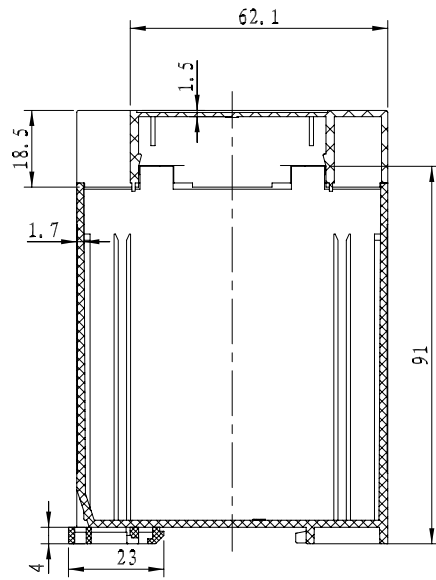
剖面 B-B
