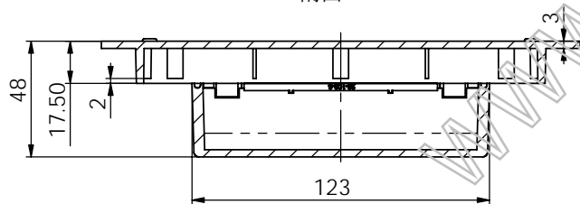
剖面 B-B
