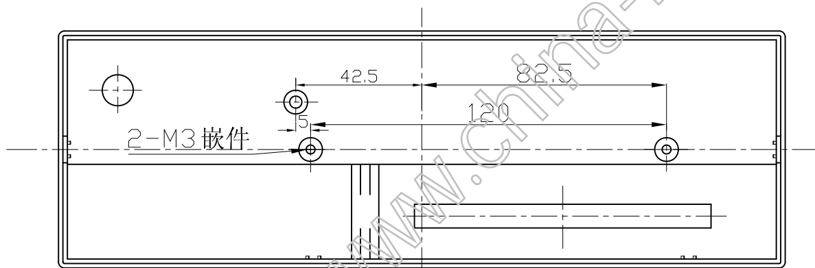
上盖底视图
