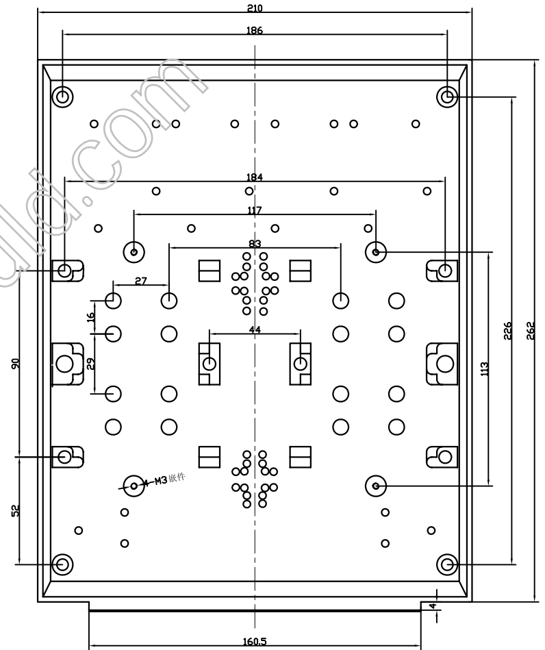
下盖正视图
