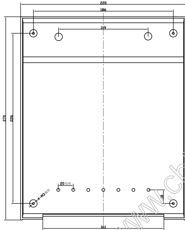
上盖反视图
