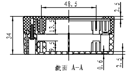
截面 A-A
