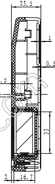
截面 A-A
