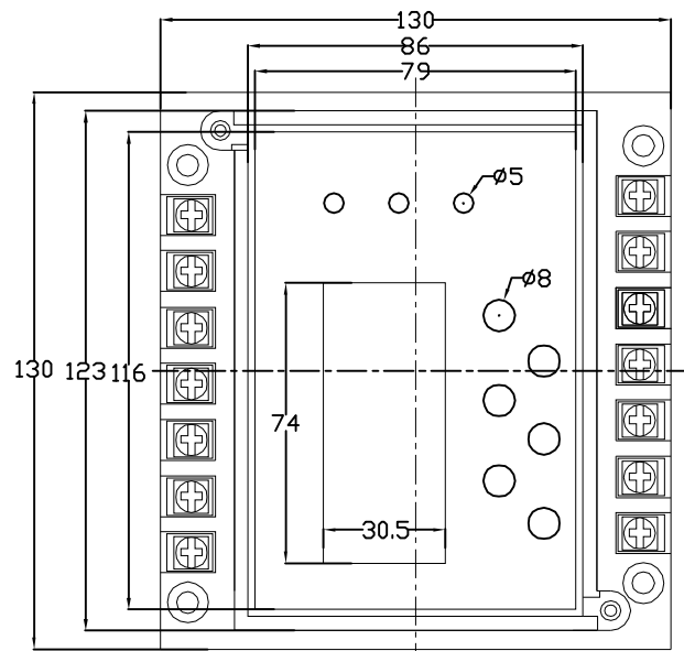
下盖正视图
