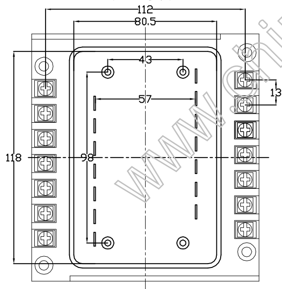
下盖正视图
