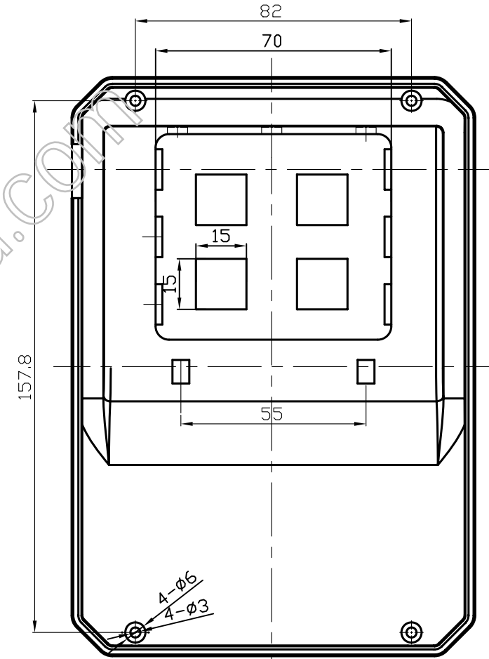
下盖正视图
