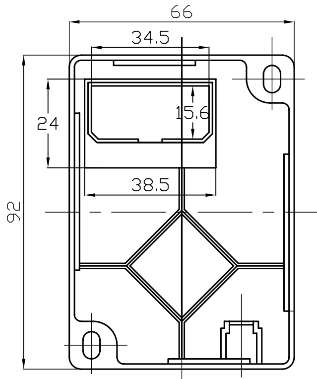
下盖主视图
