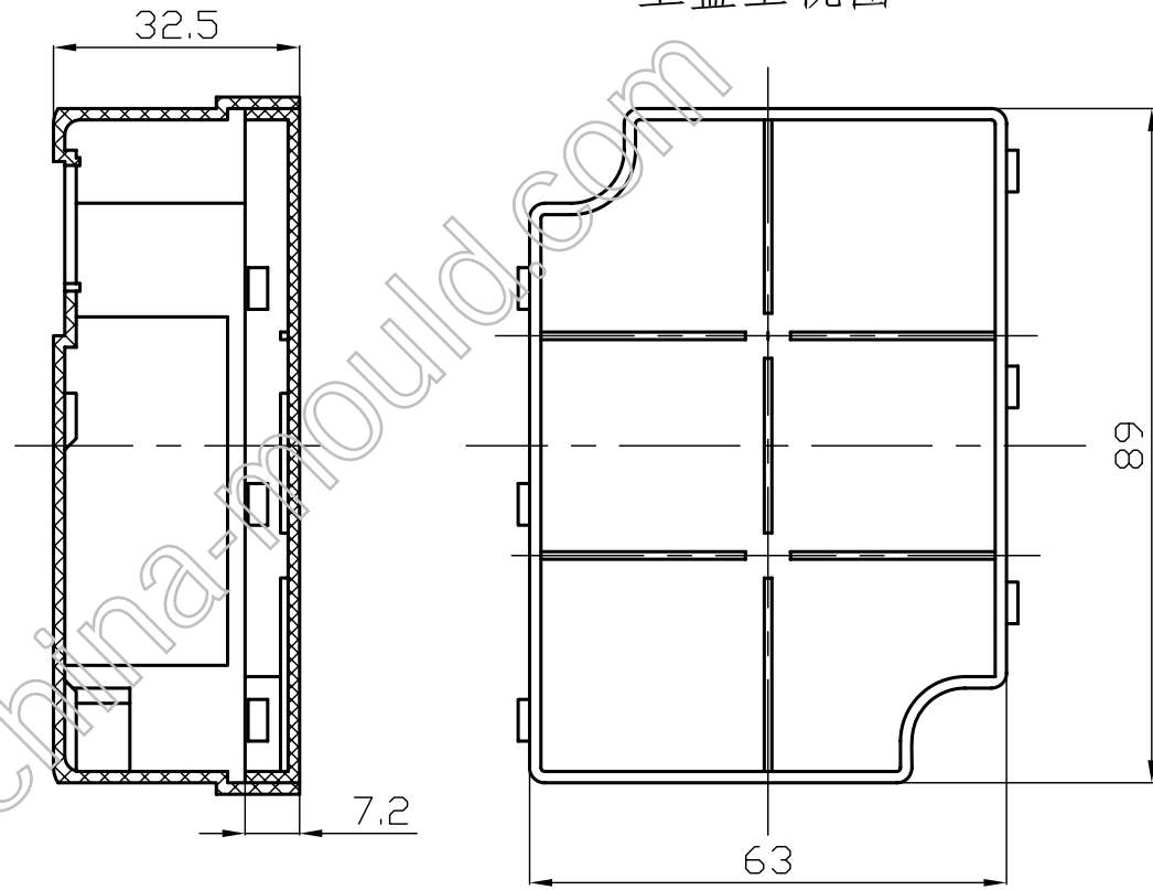
上盖主视图
