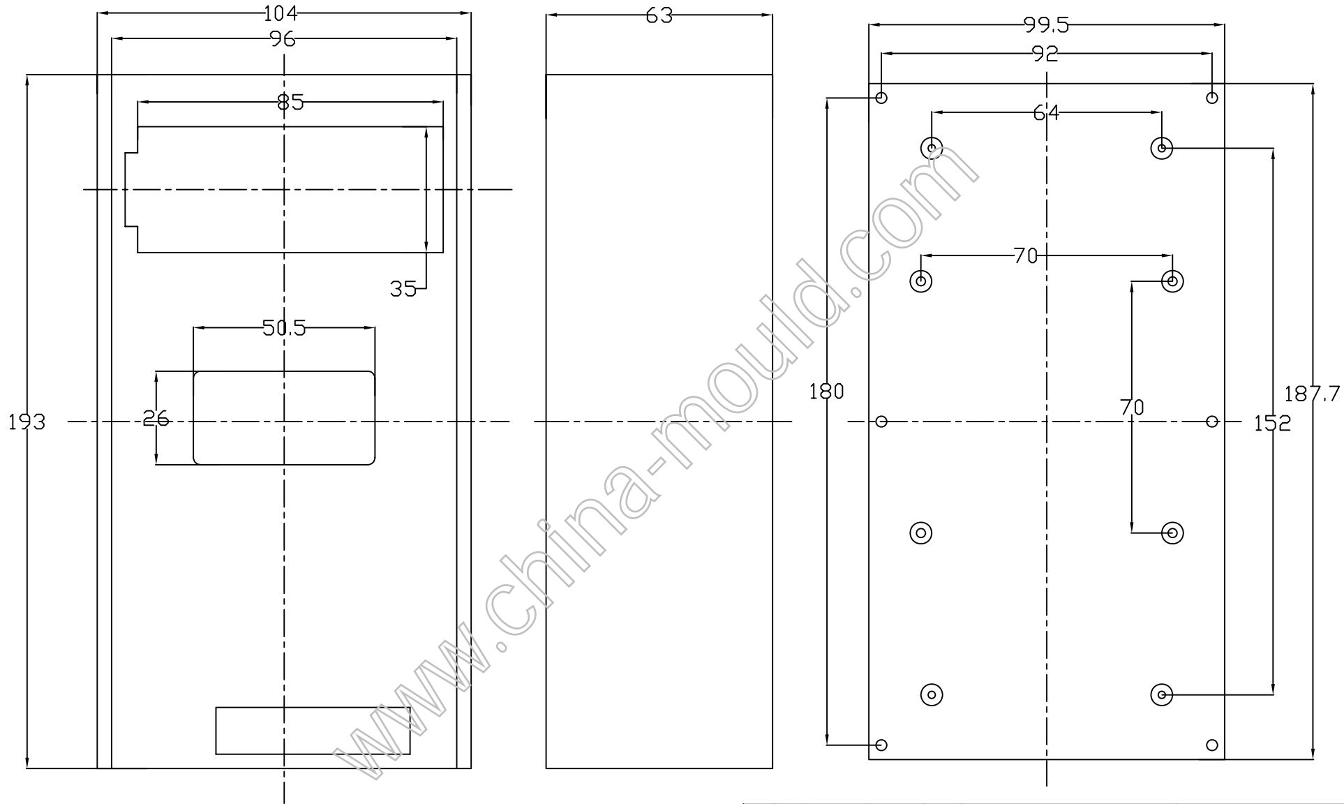
下盖板底视图
