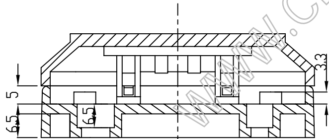
B-B
