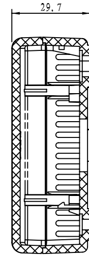
剖面 A-A
