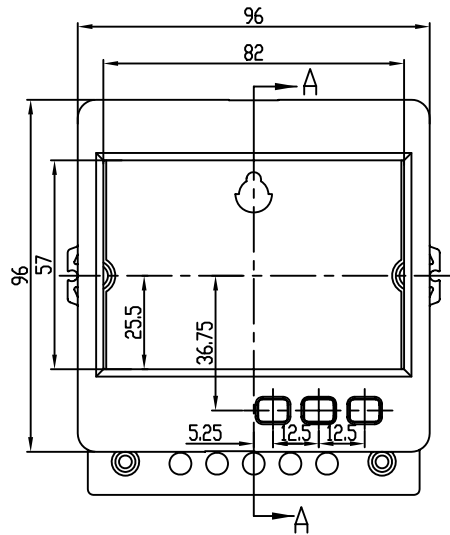
塑料底座平面图
