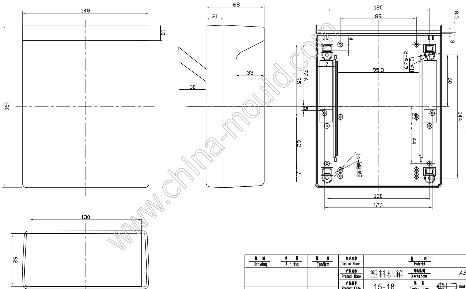
下盖正视图
