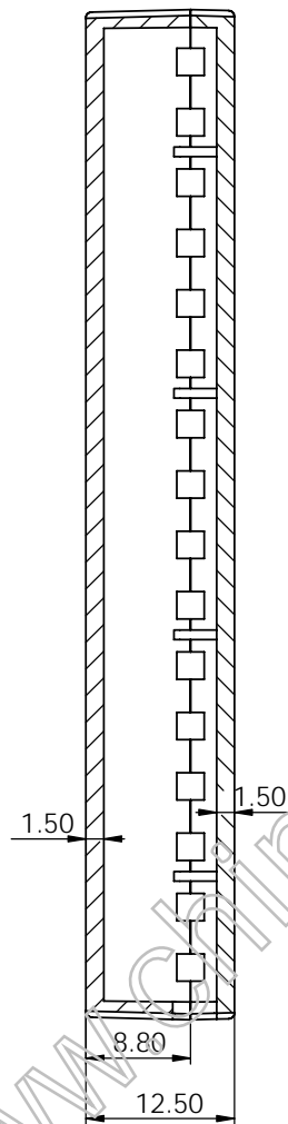
剖面 A-A
