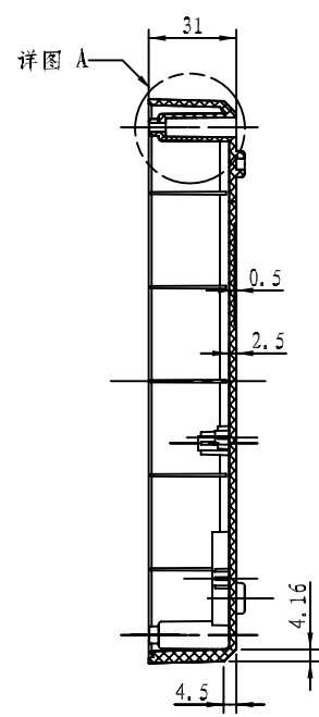
剖面 A-A
