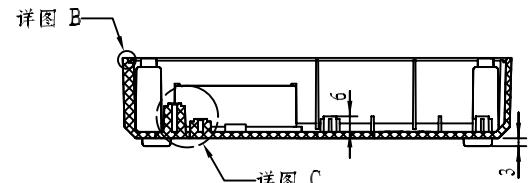
剖面 B-B
