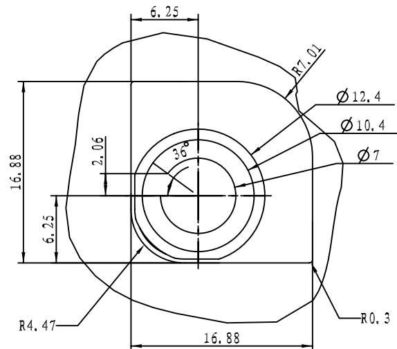
细节 B 比例 3:1
