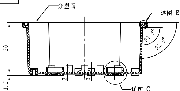
剖面 A-A
