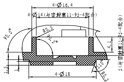
细节 C 比例 3:1
