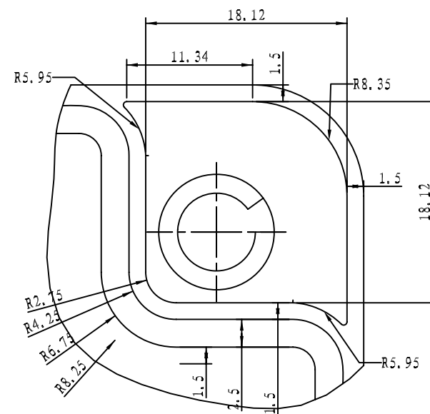
细节 D 比例 3:1
