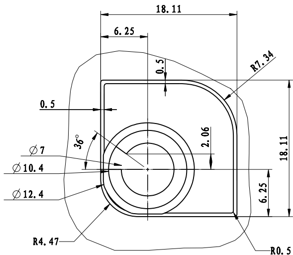
细节 B 比例 3:1
