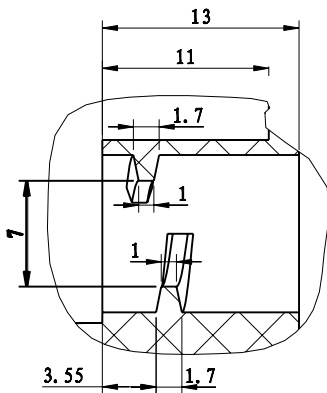
细节 D 比例 3:1
