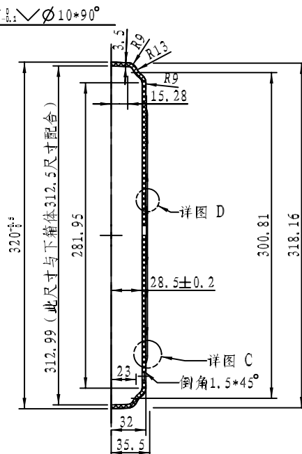
剖面 A-A
