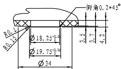
细节 B 比例 1:1
