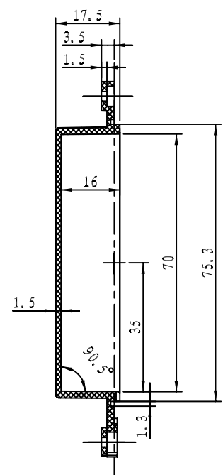
剖面 A-A
