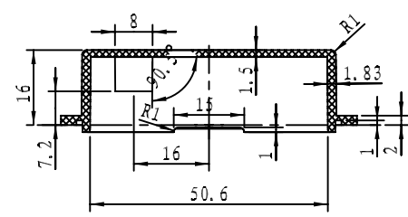
剖面 B-B
