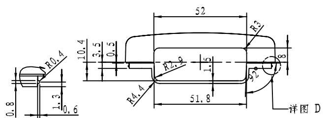
细节 D 比例 7:5
