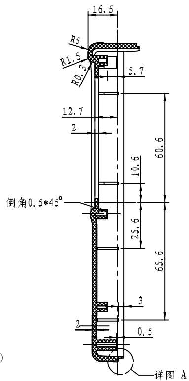
剖面 A-A
