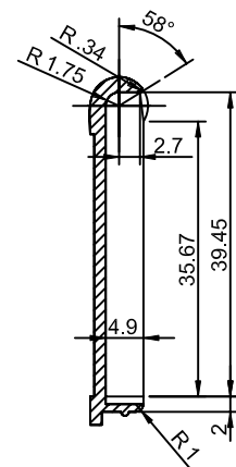
剖面 A-A
