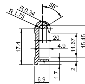
剖面 A-A
