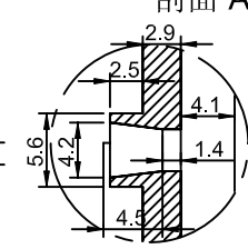
局部放大视图 F
