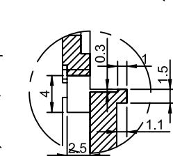
局部放大视图 E
