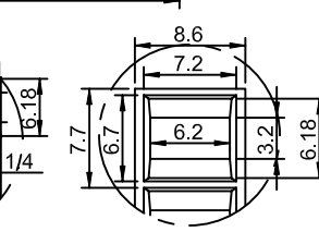
局部放大视图 I
