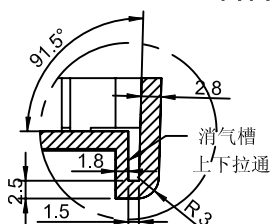
局部放大视图 C
