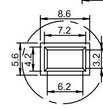
局部放大视图 G
